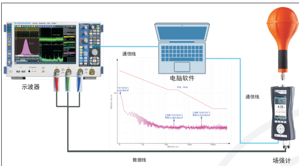
系统原理图
